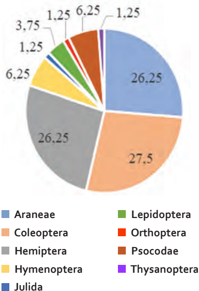
Figura 3. Percentagem de exemplares das diferentes ordens de artrópodes coletadas no BioBlitz Açores 2023, no Jardim Duque da Terceira.
